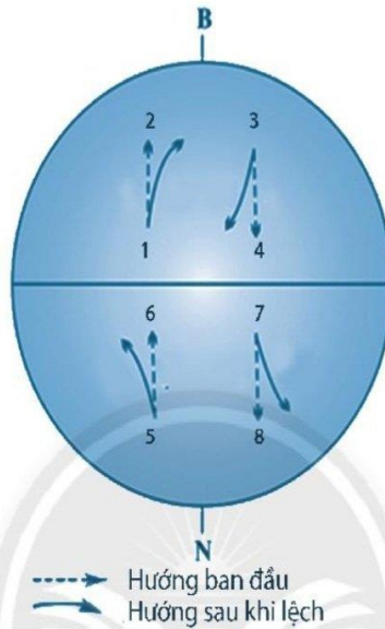
Hình 6.2. Sự lệch hướng do vận động tự quay của Trái Đất
