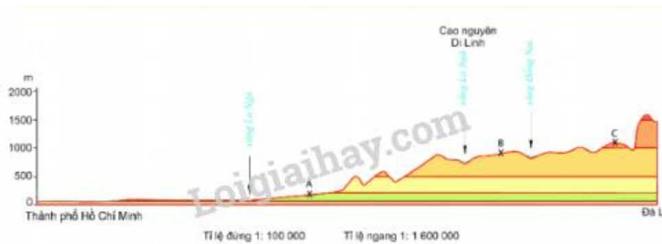
Hình 11.3. Lát cắt địa hình từ Thành phố Hồ Chí Minh đến Đà Lạt.
